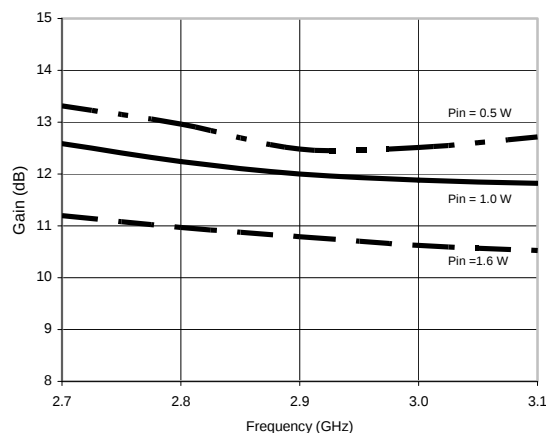
ILT2731M15 : 100us / 10% / 28V / Idq=10mA
